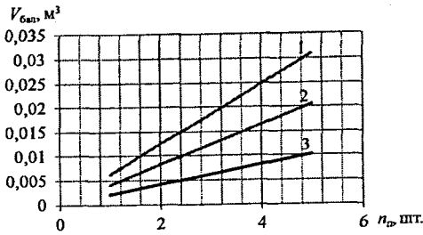
Рисунок 3 – Зависимость объема баллона V_{\text{бал}} от количества подкачек n_p при давлении P_{\text{бал}} = 1,0 МПа
