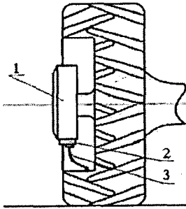
Рисунок 1 – Общий вид установки на колесе регулятора давления воздуха в шинах колесных машин
