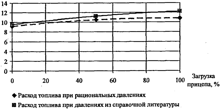
Рисунок 7 – Зависимость изменения расхода топлива от загрузки прицепа при движении по сухой твердой опорной поверхности
