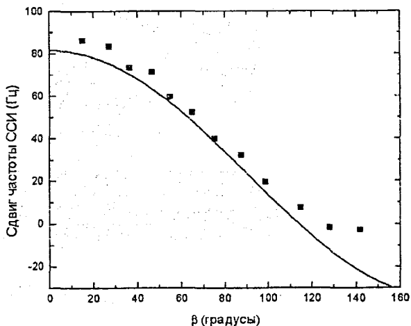
Рис. 6. Зависимость сдвига частоты от ларморовской в импульсном ЯМР для смеси «с-состояния» и «f-состояния» из работы [10]. Точки – экспериментальные данные, полученные при давлении 29,3 бар, в магнитном поле 224 Э и при температуре 0,82T_{ca}^* . Сплошная кривая – теоретическая (подробности см. в тексте).
