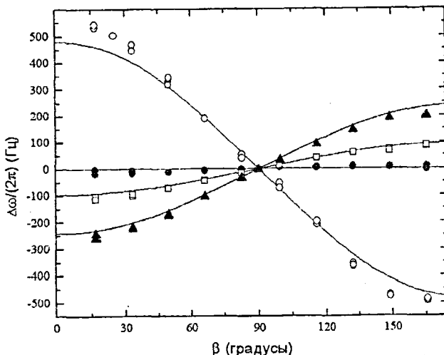
Рис.4 Зависимость сдвига частоты ССИ от ларморовской от угла отклонения намагниченности \beta в А-подобной фазе в OG-SG состоянии. Образец №2. (○) - \mu = 0 ; (●) - \mu = \mu_{c2} = 54,7^\circ ; (□) - \mu = 63,4^\circ ; (▲) - \mu = 90^\circ . Частота ЯМР 341,5 кГц, T = 0,81 T_{ca}^* , давление 26 бар.
