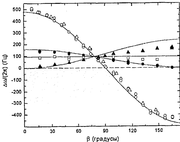
Рис.3 Зависимость сдвига частоты сигнала свободной индукции (ССИ) от ларморовской от угла отклонения намагниченности \beta в А-подобной фазе в OG-SN состоянии. Образец №2. (○) и (Δ) - \mu = 0 ; (●) - \mu = 54,7^\circ ; (□) - \mu = \mu_{c1} = 63,4^\circ ; (▲) - \mu = 90^\circ . Частота ЯМР 341,5 кГц. Данные, обозначенные (Δ), получены на частоте 664 кГц, но пересчитаны к частоте ЯМР 341,5 кГц. T = 0,81 T_{ca}^* , давление 26 бар.
