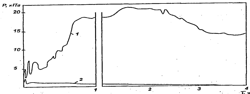
Рис. 3. 1. Давление коксования (1) и газовое давление (2) в промышленных условиях
