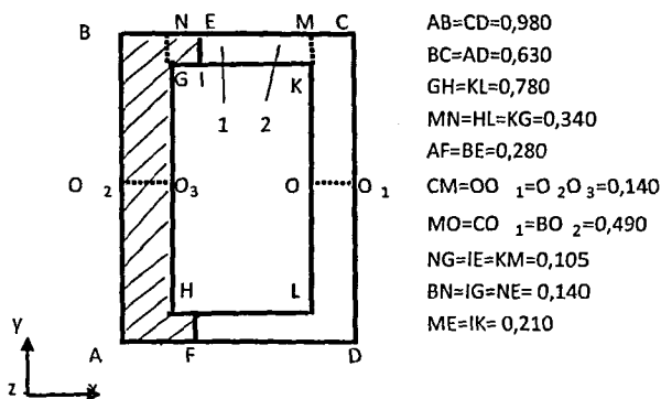
Рис. 6.2. Схема для расчета прогрева кладки
