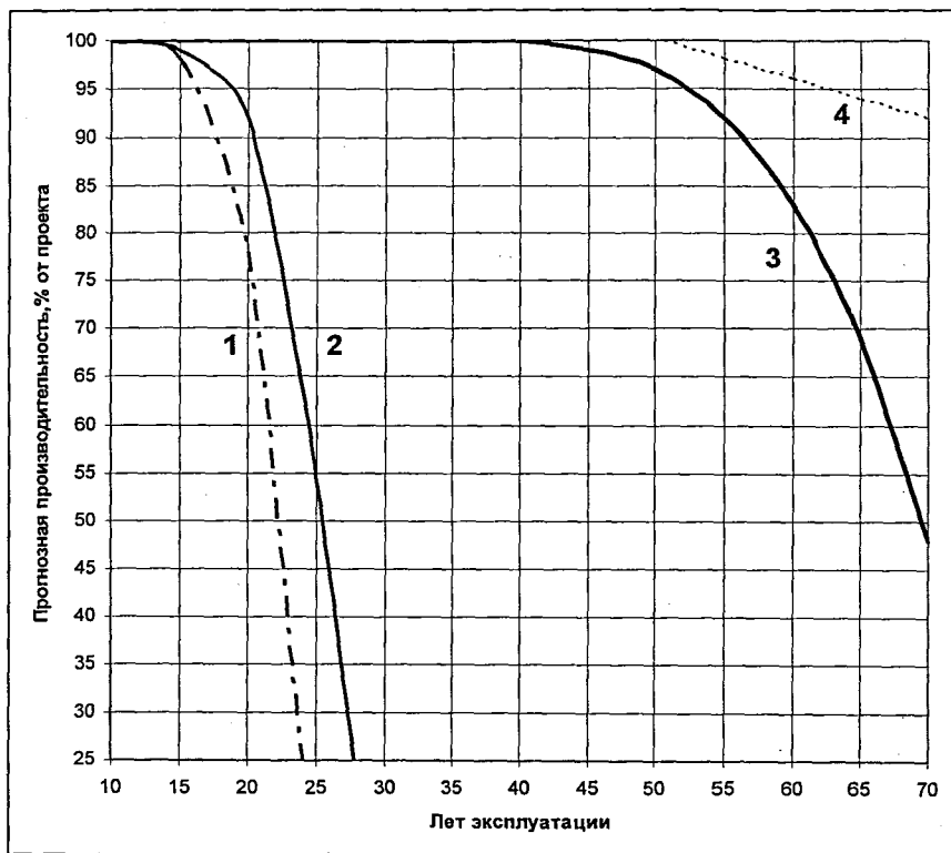
Рис 5.1 Прогнозная производительность батарей с объемом камер 41,6 \text{ м}^3 в процессе эксплуатации по состоянию: 1- головочных участков кладки; 2 – основного массива кладки простенков по схеме нагружения «консоль»; 3 – основного массива кладки простенков по схеме нагружения «балка, защемленная с двух сторон»; 4 – кладки зон косых ходов и регенераторов.
