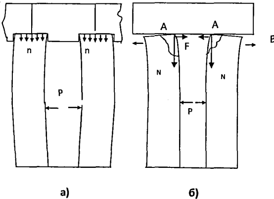
Рис. 4.2 Схемы нагружения простенков:
