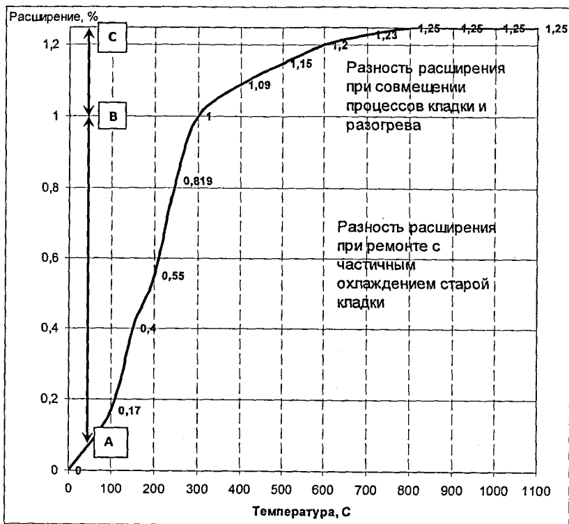
Рис. 6.1. Кривая обратимого термического расширения динаса
