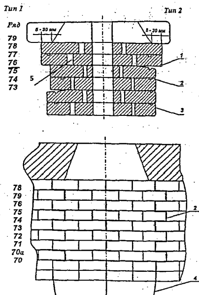
Рис. 4.3. Характеристика разрушений кладки под вторым люком коксовой батареи с объемом камер 41,3 м 3 :
