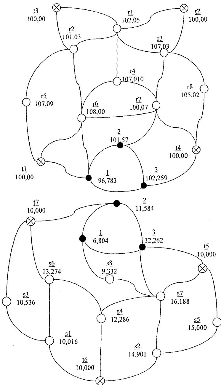
Рис. 2 – Схема нивелирных сетей
