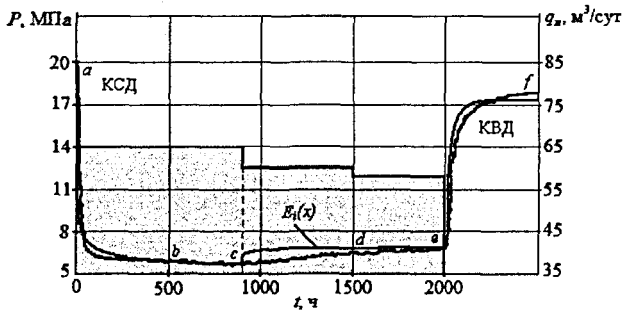
Рисунок 6 - График исследования скважины № 521 Западно-Ноябрьской
