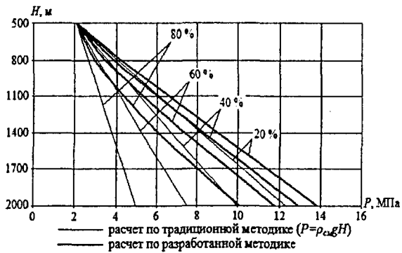
Рисунок 1 - Распределение давления в затрубном пространстве скважины при различном газосодержании (ГС, %)
