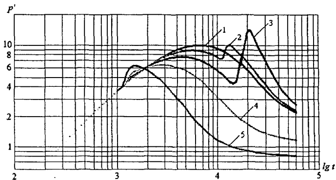
Рисунок 10 – Производные депрессии на пласт для скважин с различным профилем: 1- вертикальный ствол, 2 - 5 - искривленный с углом наклона 30^\circ , 45^\circ , 60^\circ и 75^\circ .
