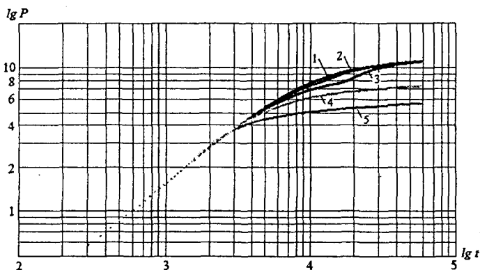
Рисунок 9 – Кривые депрессии на пласт для скважин с различным профилем: 1- вертикальный ствол, 2 - 5 - искривленный с углом наклона 30^\circ , 45^\circ , 60^\circ и 75^\circ .
