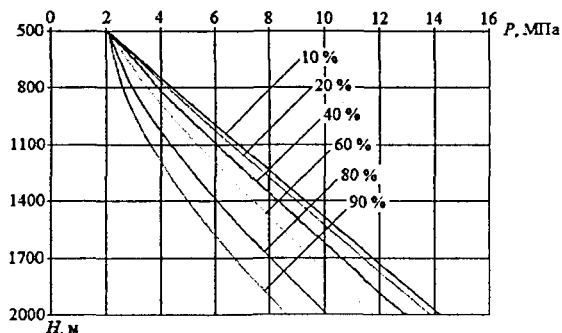
Рисунок 2 - Распределение давления в затрубном пространстве скважины по глубине при различном газосодержании (ГС, %) на H_{дин}
