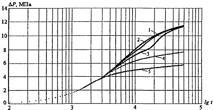
Рисунок 8 – Кривые депрессии на пласт для скважин с различным профилем: 1- вертикальный ствол, 2 - 5 - искривленный с углом наклона 30°, 45°, 60° и 75°.
