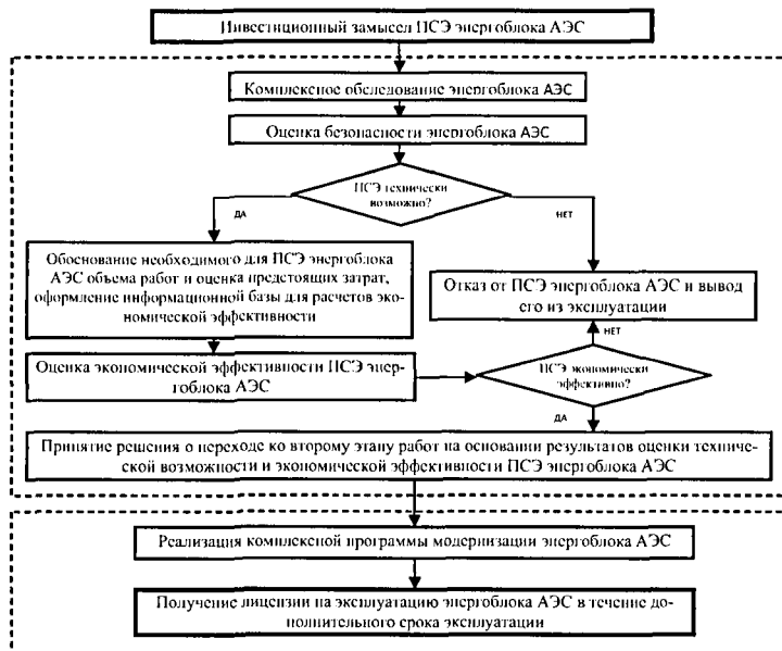
Рис. 1. Этапы реализации проекта ПСЭ энергоблока АЭС
