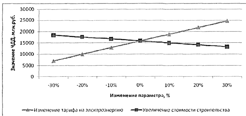
Рис. 3. Чувствительность ЧДД к изменению влияющих факторов
