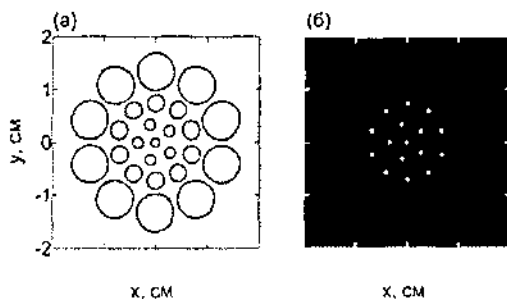
Рис. 7. Линзовый массив для одновременного образования филаментов как в центре, так и на периферии пучка (а), и филаменты, образованные этим массивом (б). Пиковая мощность импульса превышает критическую мощность самофокусировки в 100 раз. Радиус центральной линзы r_0 = 1 мм, ее радиус фокусировки 16,5 м
