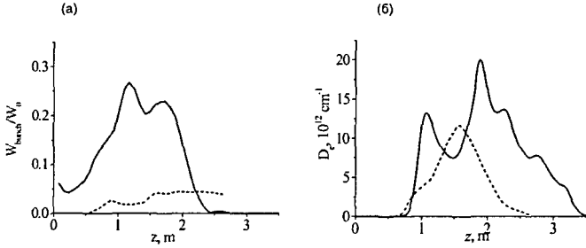
Рис. 5. (а) — энергия в области флуоресценции в зависимости от расстояния z , (б) — линейная плотность плазмы в зависимости от расстояния z . Сплошная кривая на обоих рисунках соответствует узкому длинному импульсу ( \tau_p = 200 фс, \tau_0 = 27 фс, \alpha_0 = 1 мм), штриховая — широкому короткому импульсу ( \tau_p = 100 фс, \tau_0 = 27 фс, \alpha_0 = 1.5 мм)
