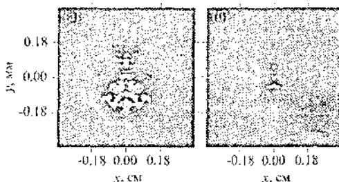
Рис. 2. Пространственные распределения плотности энергии излучения суперконтинуума (а) в коротковолновой части спектра (750 нм), (б) — в длинноволновой (850 нм). Центральная длина волны составляет 800 нм, энергия импульса — 5 мДж, его длительность — 27 фс
