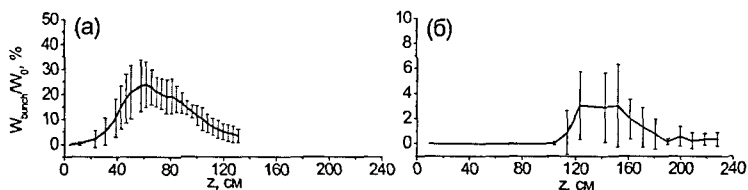
Рис. 3. Средняя по 12 реализация распределений интенсивности на выходе лазерной системы энергия, локализованная в области флуоресценции. (а) соответствует филаментации пучка меньшего диаметра, (б) — большего диаметра. Центральная длина волны составляет 800 нм, энергия импульса — 7 мДж, его длительность — 27 фс
