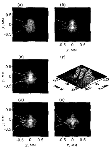
Рис. 1. Поперечные распределения плотности энергии на различных расстояниях z : (а) — z = 0 (начальное распределение), (б) — z = 7.5 см независимое развитие двух «родительских» филаментов, (в, г) — z = 11.2 см рождение «дочернего» филамента, как результат взаимодействия кольцевых структур «родительских» филаментов, (д) — z = 16.9 см начало «умирания» верхнего филамента, (е) — z = 20.6 см «гибель» верхнего филамента. Пиковая мощность превышает критическую мощность самофокусировки в 8 раз, длительность импульса 27 фс
