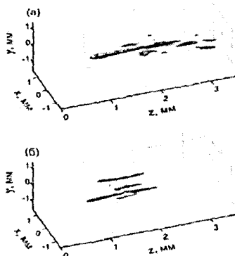
Рис. 4. Плазменные каналы многих филаментов в рассматриваемой модельной среде с увеличенной дисперсией (а) узкого длинного импульса ( \tau_p = 200 фс, \tau_0 = 27 фс, a_0 = 1 мм), (б) широкого короткого импульса ( \tau_p = 100 фс, \tau_0 = 27 фс, a_0 = 1.5 мм). Наиболее протяженный и широкий канал соответствует случаю (а)
