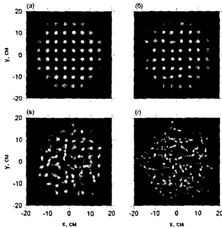
Рис. 6 Филаменты при различных значениях структурной функции атмосферной турбулентности C_n^2 . (а) соответствует C_n^2 = 7.9 \cdot 10^{-17} \text{ см}^{-2/3} , (б) — C_n^2 = 7.9 \cdot 10^{-16} \text{ см}^{-2/3} , (в) — C_n^2 = 7.9 \cdot 10^{-15} \text{ см}^{-2/3} , (г) — C_n^2 = 7.9 \cdot 10^{-14} \text{ см}^{-2/3} . Пиковая мощность импульса превышает критическую мощность самофокусировки в 100 раз. Радиус пучка составляет a_0 = 16 см, поперечный размер линзы d = 4 см, фокусное расстояние линзы R_f = 7.5 км. При переходе от (а) к (г) последовательно теряется качество регуляризации множественной филаментации в турбулентной атмосфере при использовании линзового массива
