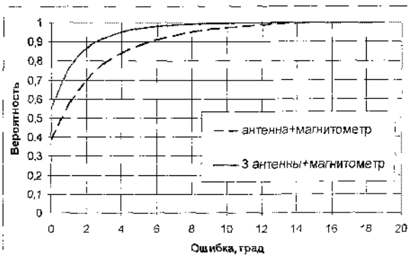
Рисунок 4 – Вероятность F(\delta_y \leq \delta) невыполнения ошибки оценки угла тангажа заданной величины ( i=63^\circ , h=300 км)
