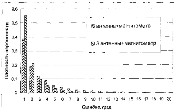
Рисунок 5 – Плотность распределения вероятности ошибки оценки угла тангажа ( i=63^\circ , h=300 км)
