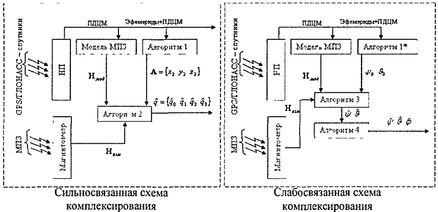
Рисунок 3 – Схемы комплексирования магнитометрических и спутниковых радионавигационных измерений
