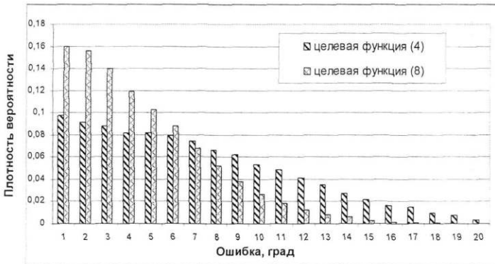
Рисунок 2 – Плотность распределения вероятности ошибки оценки угла тангажа ( i=63^\circ , h=300 км)
