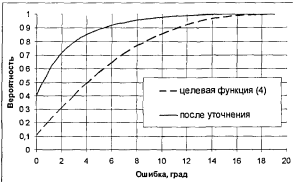
Рисунок 6 – Вероятность F(\delta_g \leq \delta) неперевышения ошибки оценки угла тангажа заданной величины ( i=63^\circ, h=300 км)
