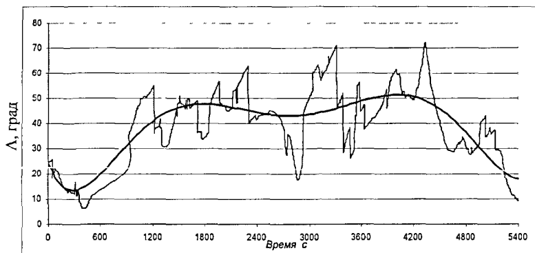
Рисунок 8 – Угол \Lambda между продольной осью КА и осью OY_2 Время T=0 соответствует 13 25 54 UTC 04 06 05
