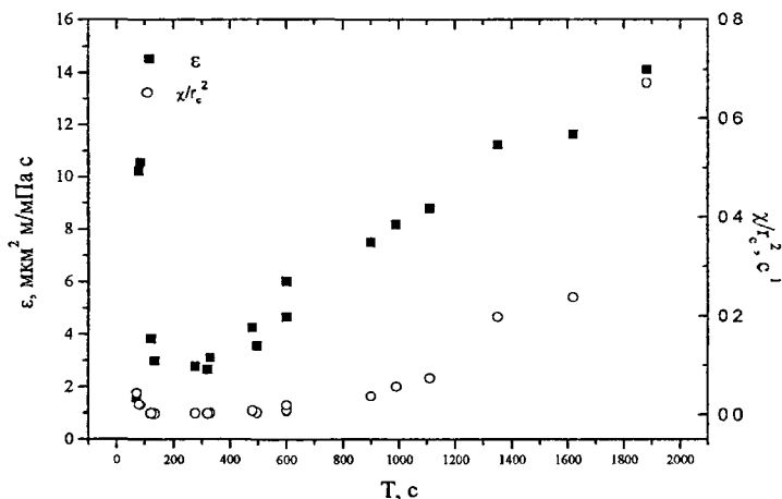
Рис 3 Расчетные значения гидропроводности \epsilon и параметра \chi/r_c^2 с учетом поправок в зависимости от периода колебаний дебита
