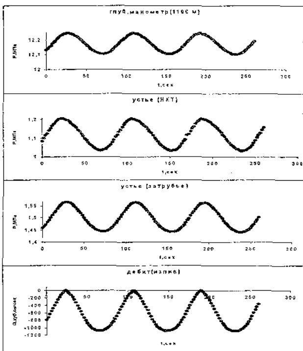
Рис.2. Пример одновременного измерения дебита и давления.
