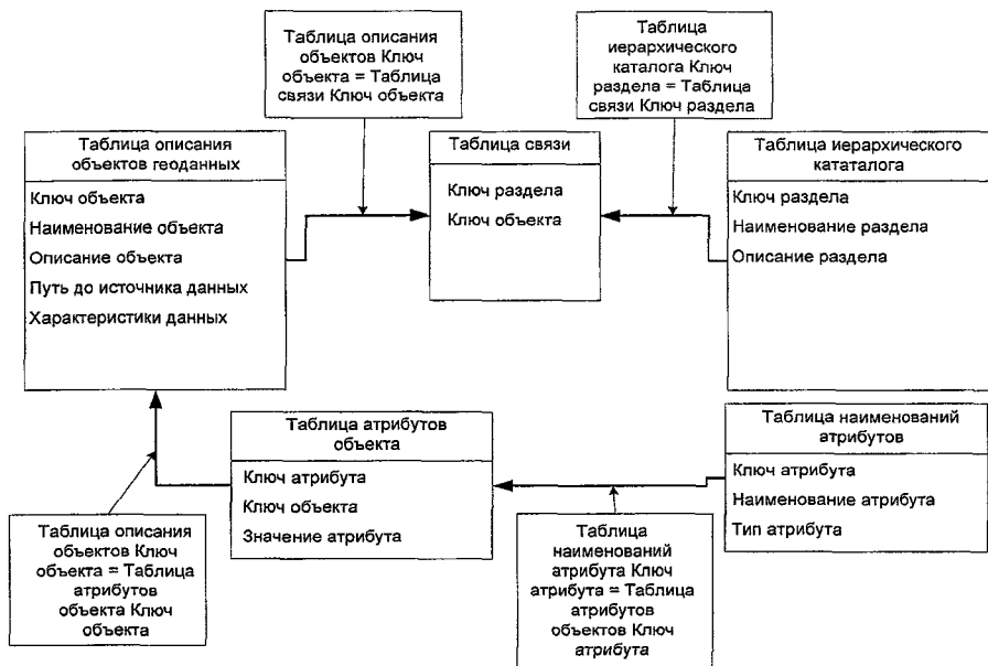
Рис 1 1 Структура таблиц каталога метаданных
