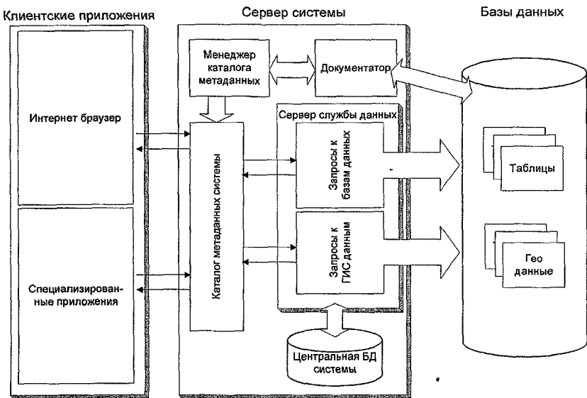
Рис 1 7 Архитектура системы
