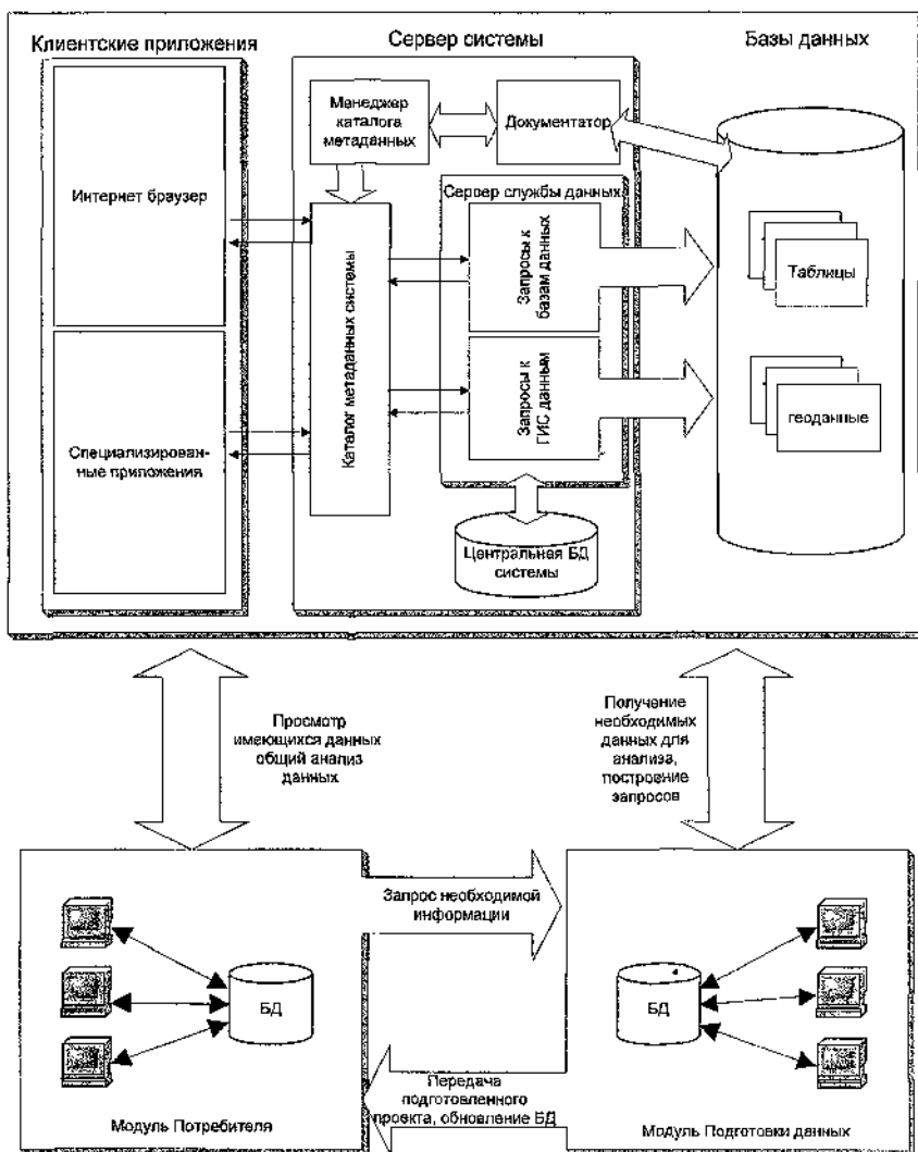
Рис. 1.9. Функциональная схема эксплуатации базы геоданных
