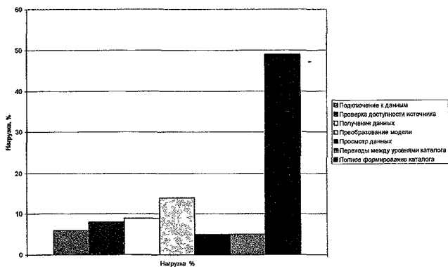
Рис 1.11 Загрузка процессора
