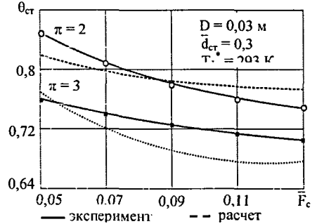
Рис. 6. Зависимость относительной температуры стержня от относительной площади сопла
