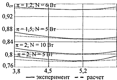
Рис. 9. Зависимость температуры стержня от диаметра диффузора
