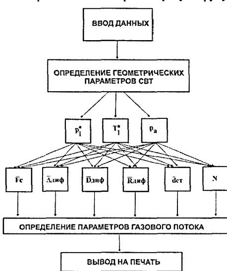
Рис. 1. Схема определения параметров газового потока с использованием ЭВМ
