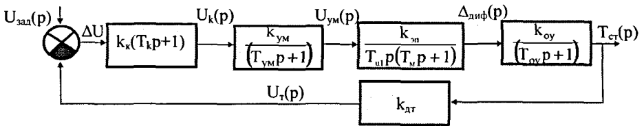
Рис. 14. Структурная схема ВСТ с корректирующим звеном
