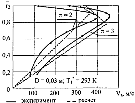
Рис.10. Распределение тангенциальной скорости по радиусу СВТ
