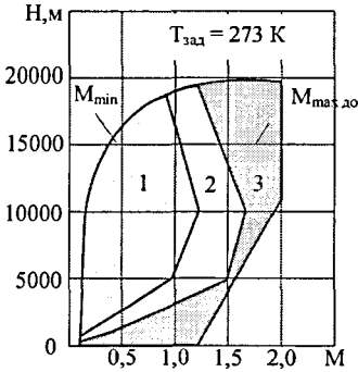
Рис. 16. Диапазон работы ВСО “Вихрь”: 1 - однокаскадной с СВТ; 2 - двухкаскадной с СВТ и ДВТ; 3 - диапазоны режимов полета ЛА
