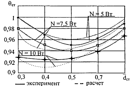
Рис. 8. Зависимость относительной температуры стержня от относительного диаметра стержня
