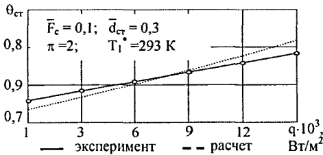
Рис. 5. Зависимость относительной температуры стержня от тепловой нагрузки
