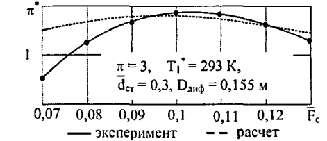
Рис. 4. Зависимость полной степени расширения от относительной площади сопла
