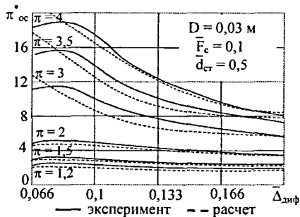
Рис. 11. Зависимость степени расширения в вихре от ширины зазора в диффузоре
