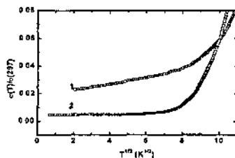
Рис. 3 Температурная зависимость проводимости одного из образцов группы В при низких температурах до отжига (1) и после (2)
