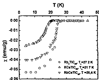
Рис. 1 Температурные зависимости магнитной восприимчивости тройных гетерофуллеридов состава KCsTlC_{60} и RbCsTlC_{60} . Также показана зависимость \chi(T) для Rb_2TlC_{60}
