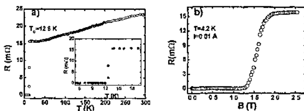
Рис. 2 Температурная (а) и магнетосолевая (б) зависимости сопротивления для образца, полученного в системе алмаз–ниобий
