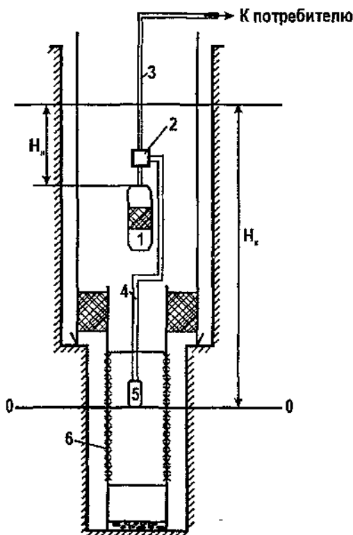
Рис 5 Расчетная схема кавитационной обработки скважины
