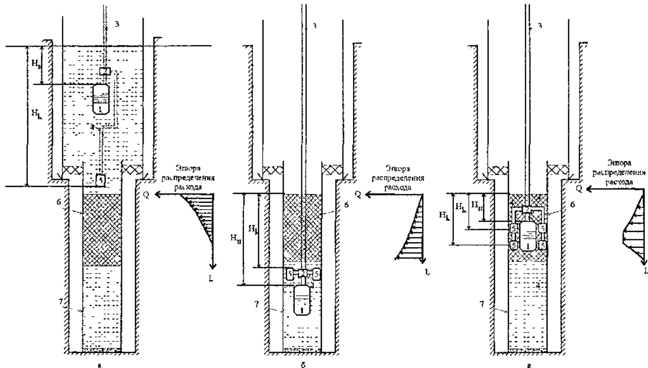
Рис 7 Рекомендуемые базовые технологические схемы установки погружных насосов и размещения кавитационных генераторов а – напорный водоносный горизонт, б – безнапорный водоносный горизонт, в – безнапорный водоносный горизонт, представленный скальными трещиноватыми горными породами 1 – погружной насос, 2 – электрогидравлический клапан, 3 – водоподъемная линия, 4 – подводная магистраль, 5 – кавитационный генератор, 6 – фильтр, 7 – отстойник H_n – глубина погружения насоса под динамический уровень ( H_n > 1м ), H_k – глубина погружения кавитационного генератора под динамический уровень
