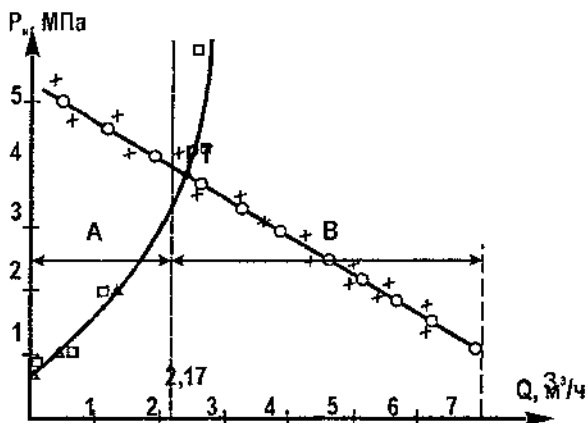
Рис. 6 Напорные характеристики погружного насоса и сети "обводная магистраль – кавитационный генератор"
