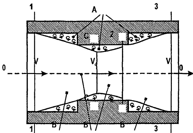
Рис 4 Расчетная схема течения жидкости в кавитационном генераторе
