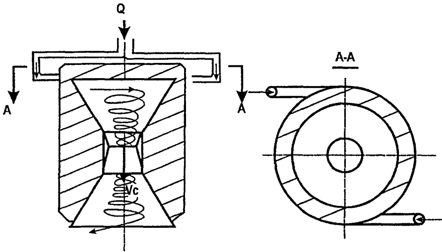
Рис 8 Центробежный кавитационный генератор
