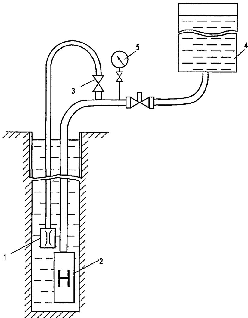
Рис 1 Схема размещения оборудования и инструмента на поверхности и в скважине для ее отработки вибратором с приводом от погружного насоса (по Меламеду Ю А и Киселеву А Т )
