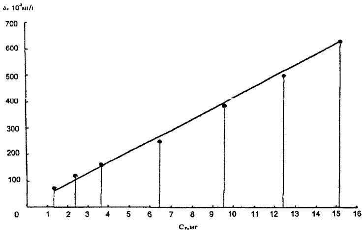
Рис 1 Изотерма адсорбции гидроксидов хрома активированным ломосиликатным адсорбентом
