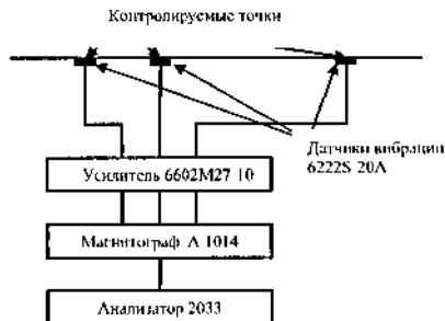
Рис 5 Схема расположения контролируемых точек на РВД и подключение приборов измерительного тракта
