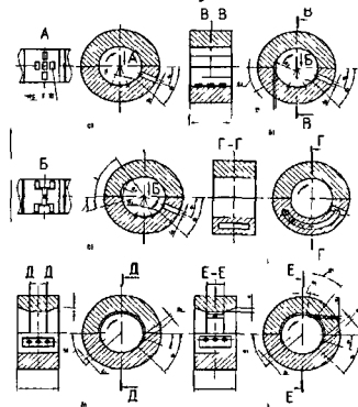
Рис 3 Варианты опытных вкладышей
