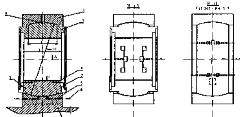
Рис 4 Конструкция штатного вкладыша для АЭС «Бушер» (K-1000-60/3000)
