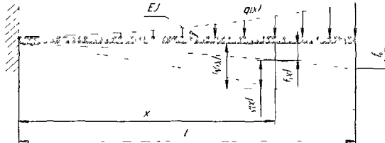
Рис 1 Расчетная схема вращающейся консольной части ротора, имеющей остаточный прогиб
