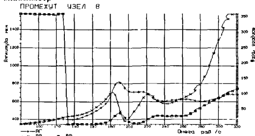
Рис. 2 АФЧХ на конце консоли имеющей начальный погиб 0,45 мм
