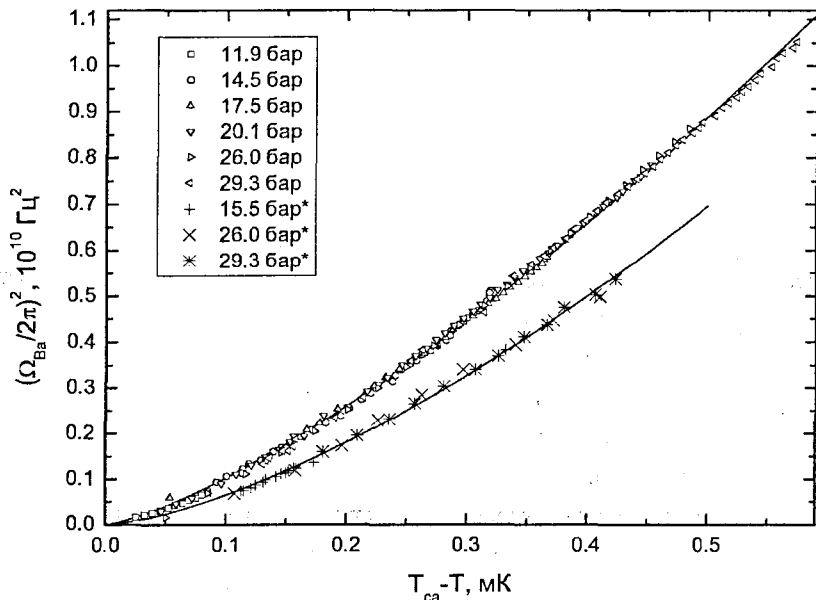
Рис. 2. Зависимость леггеттовской частоты в {}^3\text{He}-\text{V} в азрогеле от (T_{ca}-T) . T_{ca}=T_{cr}(P) соответствует давлениям, при которых были получены температурные зависимости. Зависимость имеет степенной характер \Omega_{Ba}^2 \propto (T_{ca}-T)^\alpha , \alpha \approx 1.34 . Звёздочками отмечены зависимости, измеренные нами в другом образце {}^3\text{He} в азрогеле ( \alpha \approx 1.48 ).
