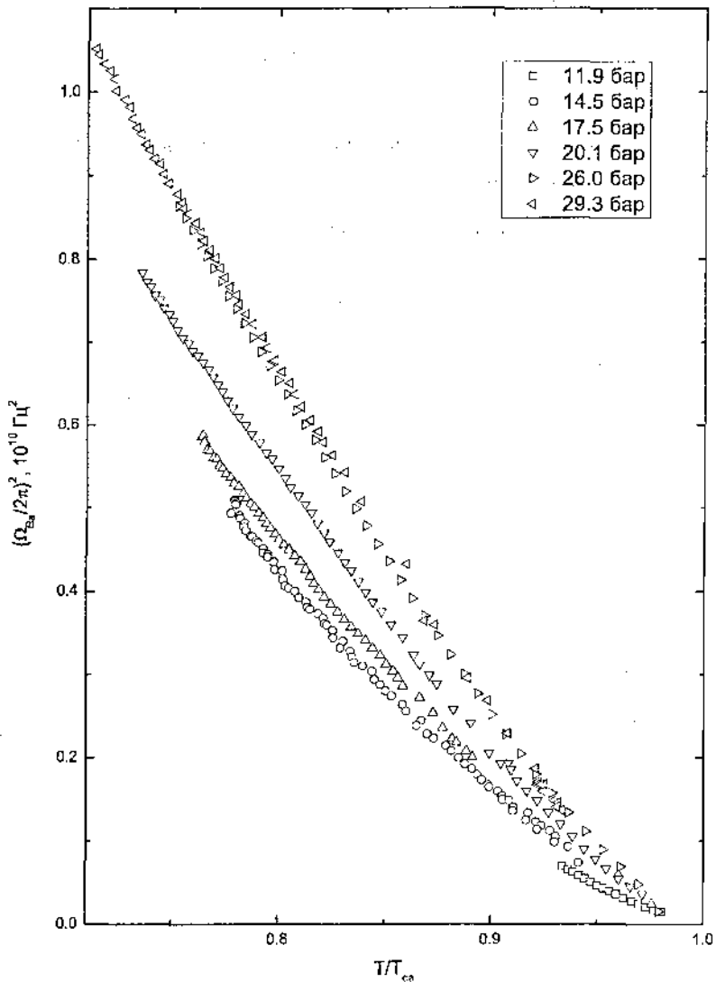
Рис. 1. Зависимость леггеттовской частоты в ^3\text{He-B} в аэрогеле от температуры при разных давлениях. T_{\text{сн}}=T_{\text{сн}}(P) — температура сверхтекучего перехода в ^3\text{He} в аэрогеле для соответствующих давлений.
