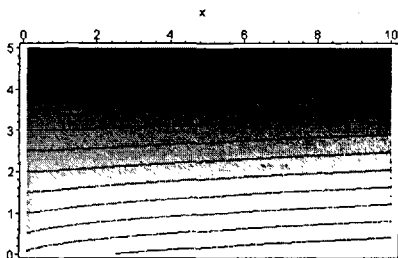
Солёность S
