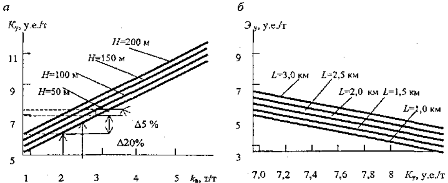
Рисунок 2 — Зависимость удельных капитальных затрат от среднего коэффициента вскрыши и глубины (а); зависимость удельных эксплуатационных затрат от капитальных и дальности транспортирования (б)
