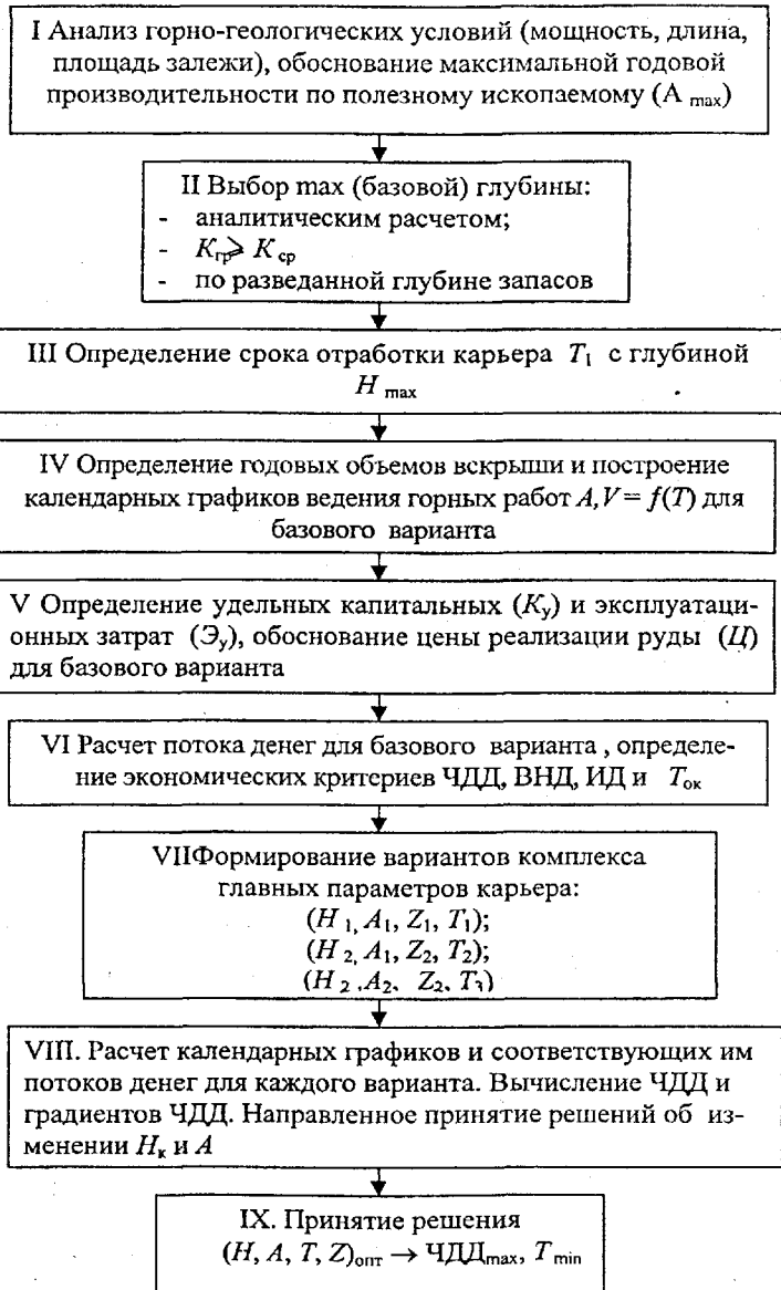
Рисунок 3 – Алгоритм определения комплекса оптимальных параметров карьера с использованием линейной стратегии принятия решений
