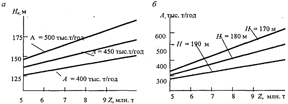
Рисунок 4 – Графики зависимости от величины запасов в контуре карьера глубины при заданной производительности по полезному ископаемому (а) и годовой производительности по полезному ископаемому при заданной глубине карьера (б).
