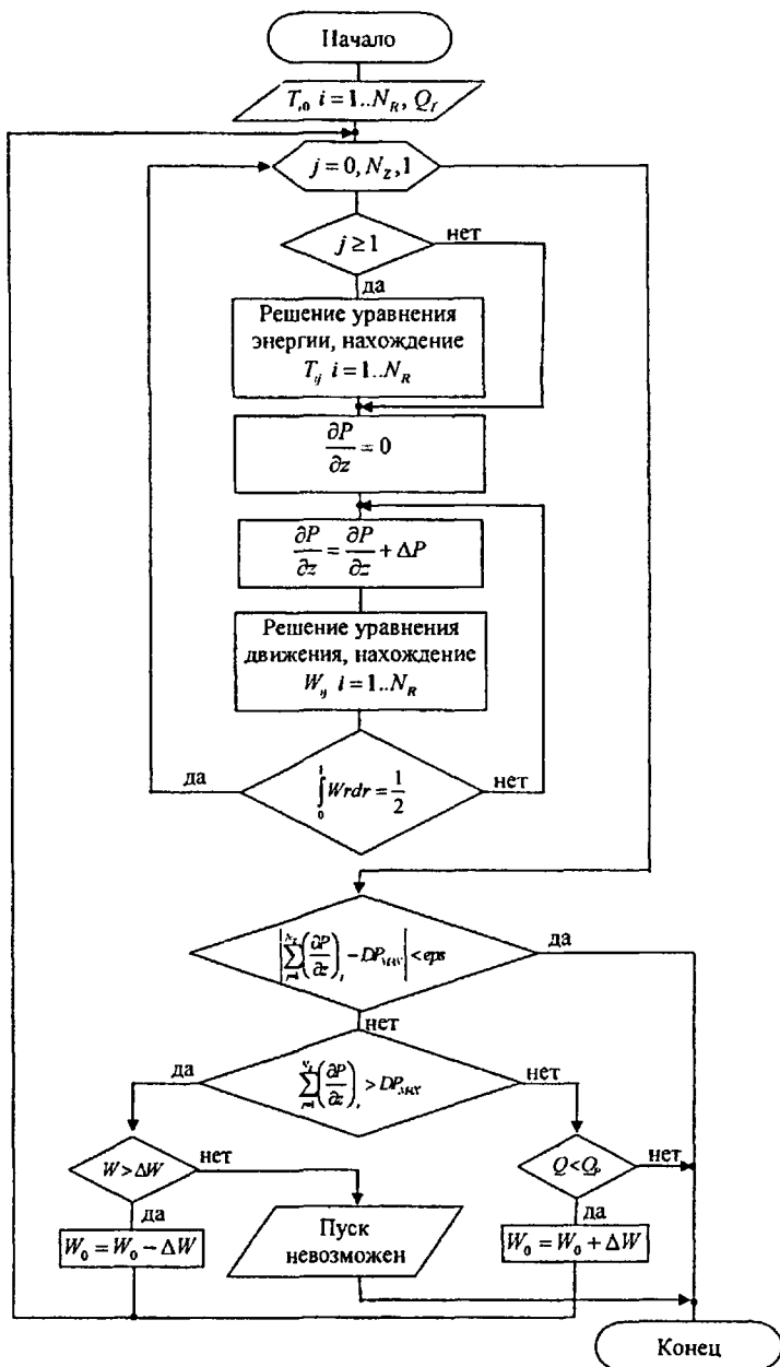
Рисунок 3 – Блок-схема моделирования нестационарного режима на слое i
