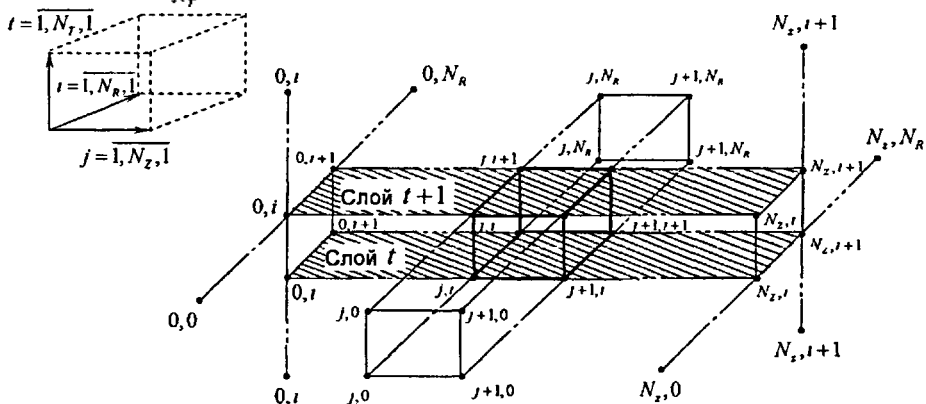
Рисунок 2 – Сеточная область решения задачи
