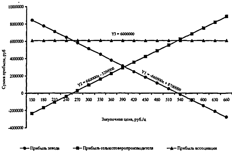
Рисунок 2 - Зависимость прибыли перерабатывающего предприятия, сельхозтоваропроизводителя и взвешенной прибыли ассоциации от закупочной цены на молоко при параметре \delta = 0.5
