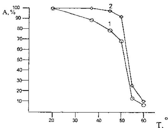
Рис. 8. Термостабильность глутамилэндопептидазы B. intermedius 1 – активность в отсутствии ионов \text{Ca}^{2+} 2 – активность в присутствии ионов \text{Ca}^{2+}
