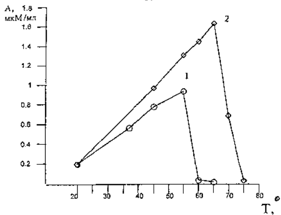
Рис. 7. Зависимость активности протеиназы B. intermedius от температуры 1 – активность в отсутствии ионов \text{Ca}^{2+} , 2 – активность в присутствии ионов \text{Ca}^{2+}
