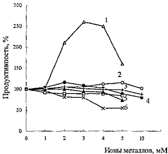
Рис.3. Влияние ионов двухвалентных металлов на биосинтез глутамилэндопептидазы B. intermedius 1 — ионы кобальта; 2 — ионы кальция; 3 — ионы марганца; 4 — ион магния; 5 — ионы меди; 6 — ионы железа; 7 — ионы цинка. За 100% принята продуктивность культуры без ионов металлов \sigma \leq 10\%
